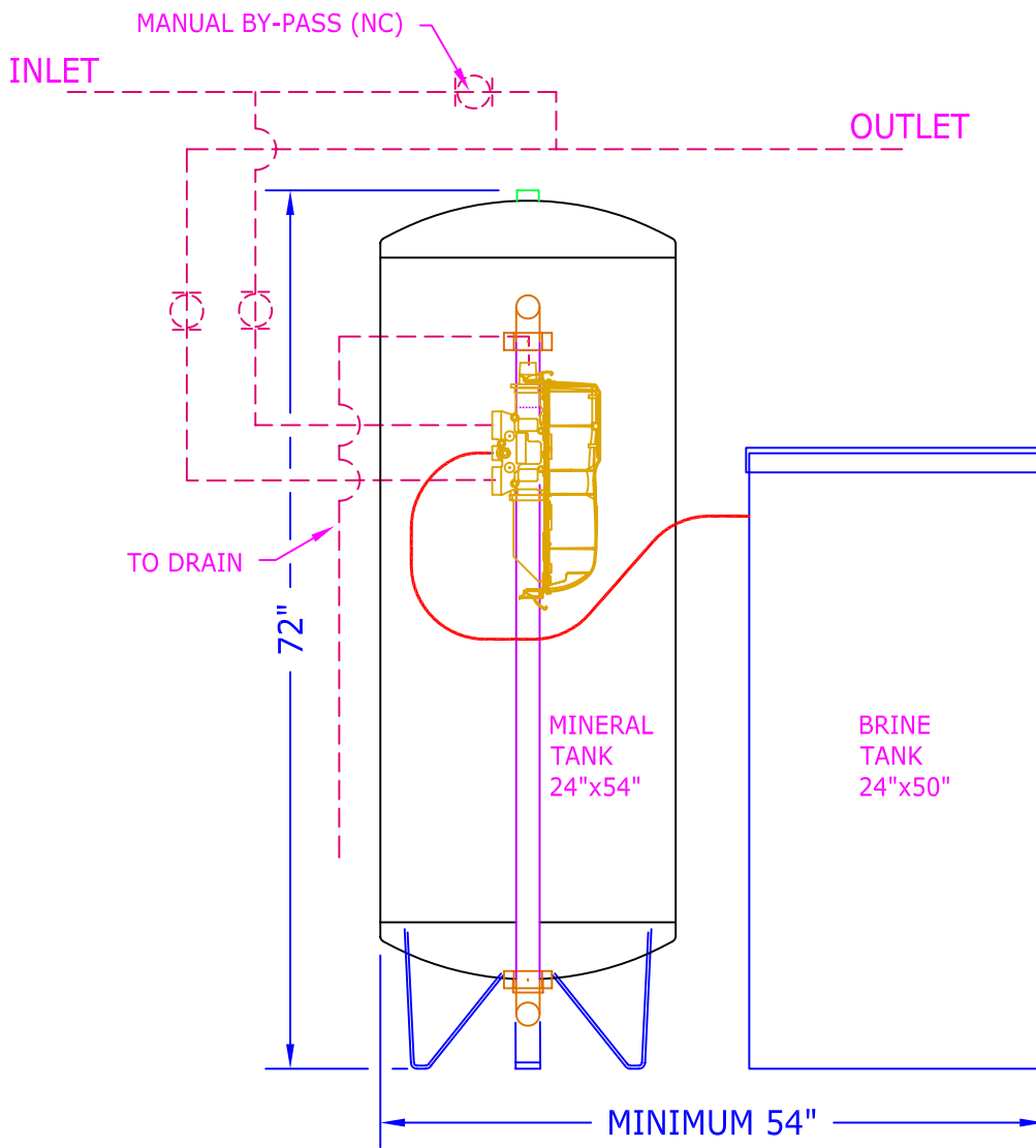
ELEVATION
