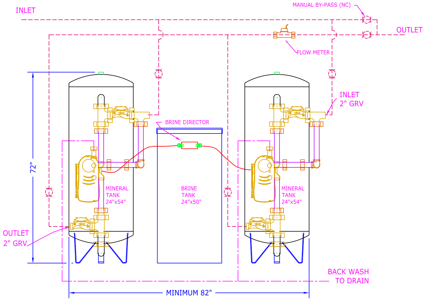
ELEVATION
