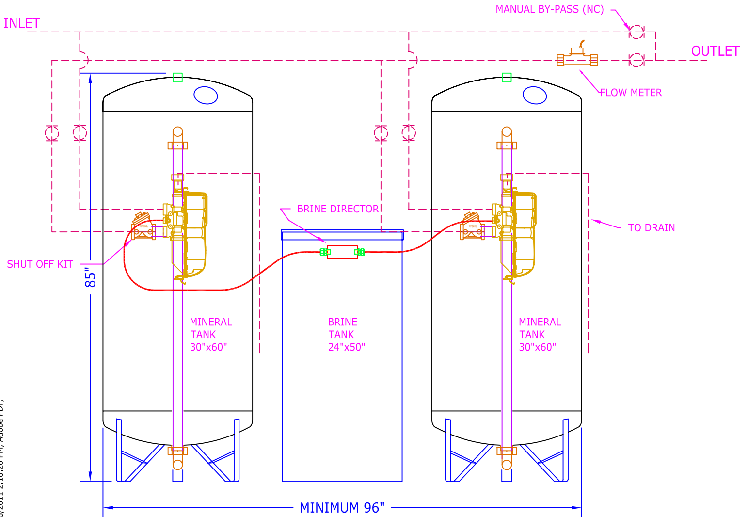
ELEVATION
