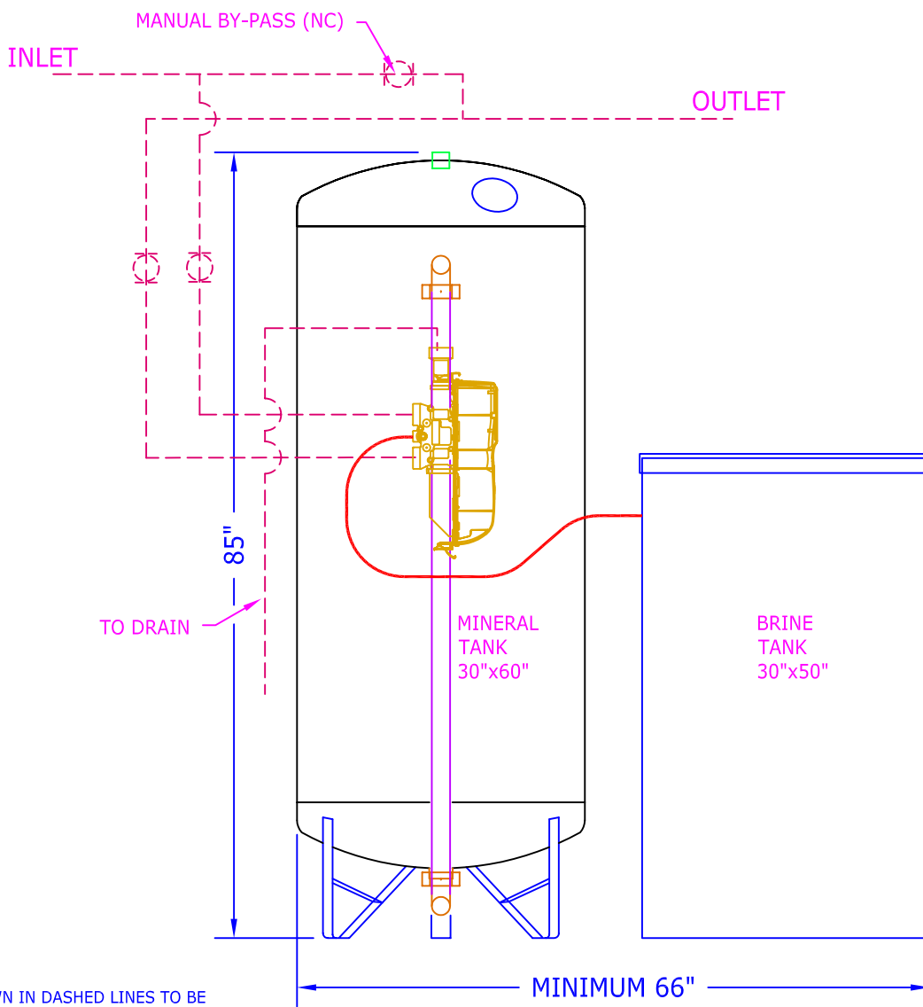
ELEVATION
