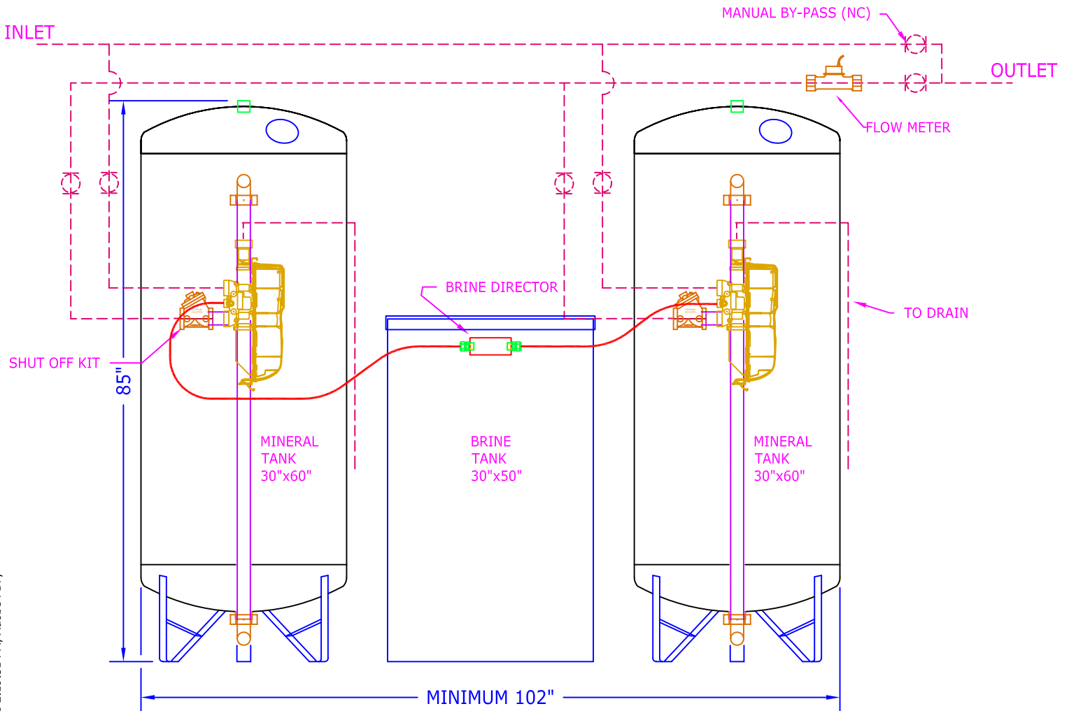
ELEVATION
