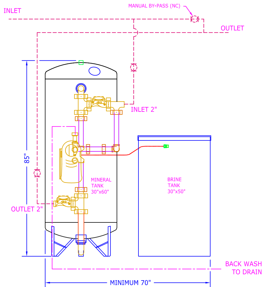
ELEVATION
