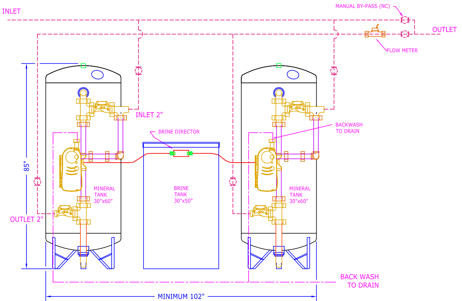
ELEVATION
