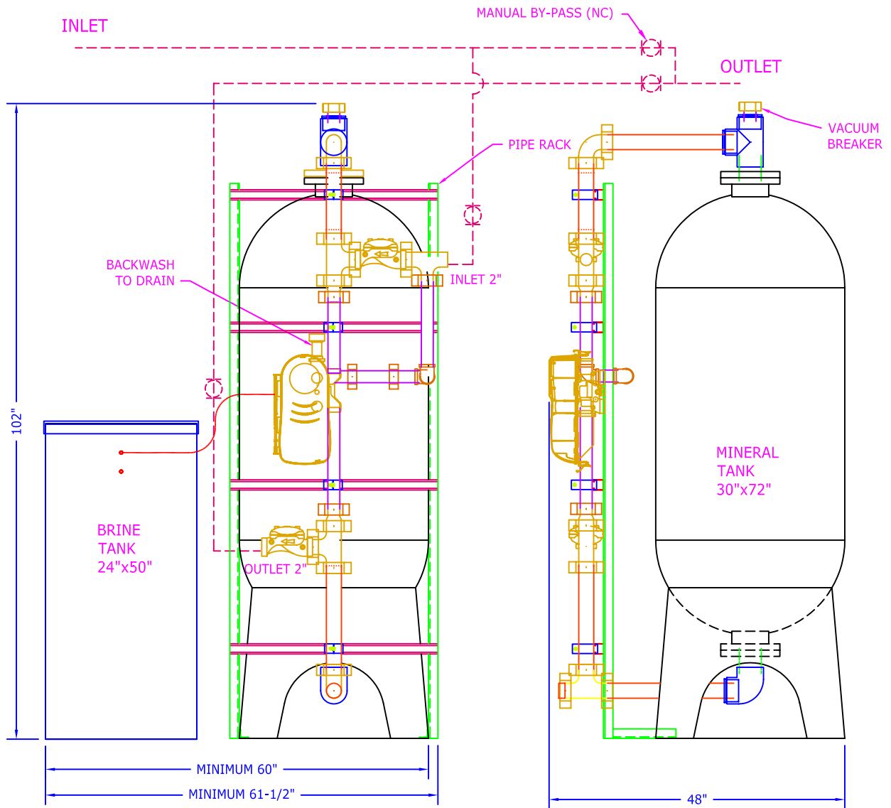
ELEVATION
