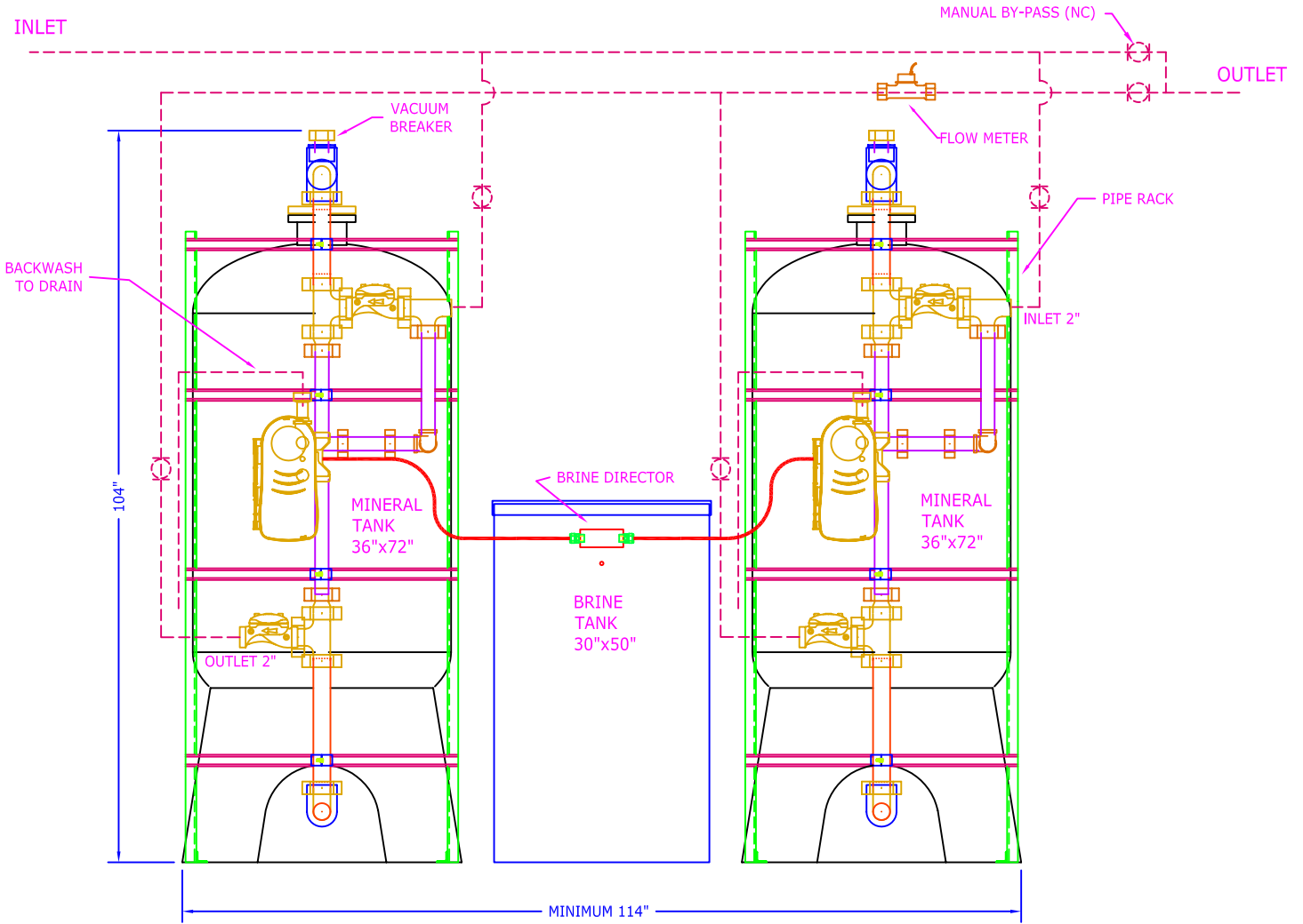
ELEVATION
