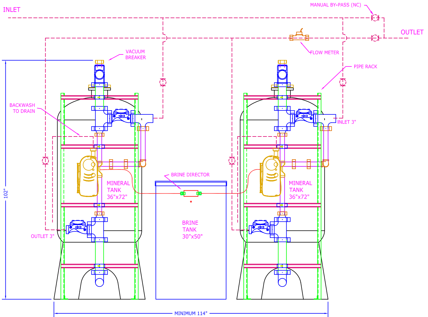
ELEVATION
