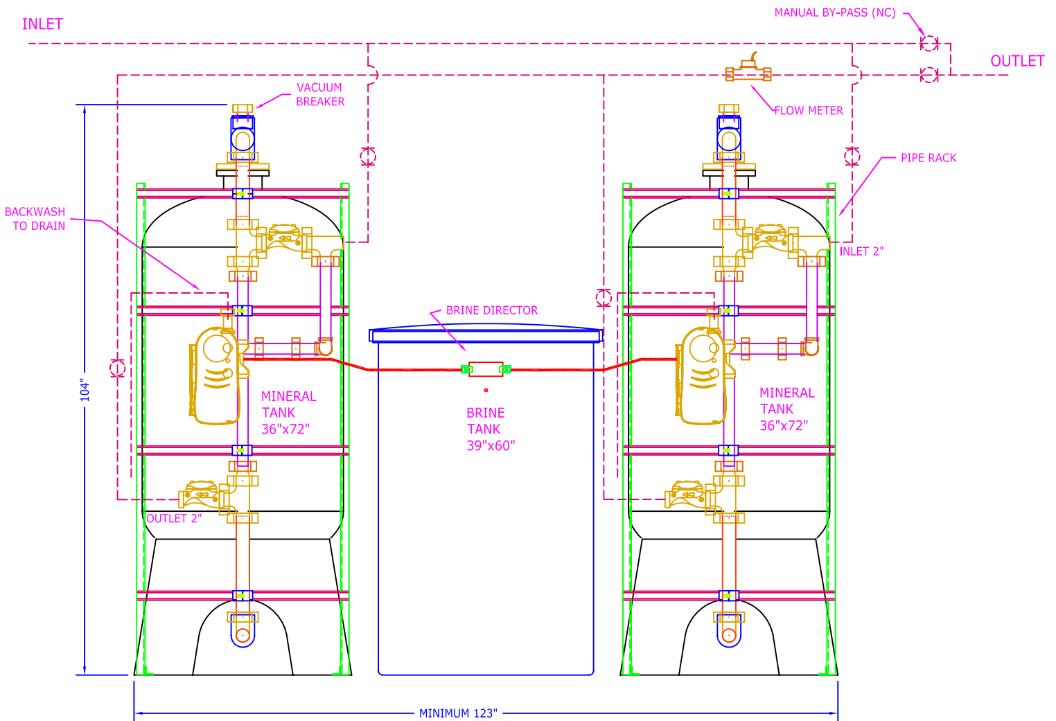
ELEVATION
