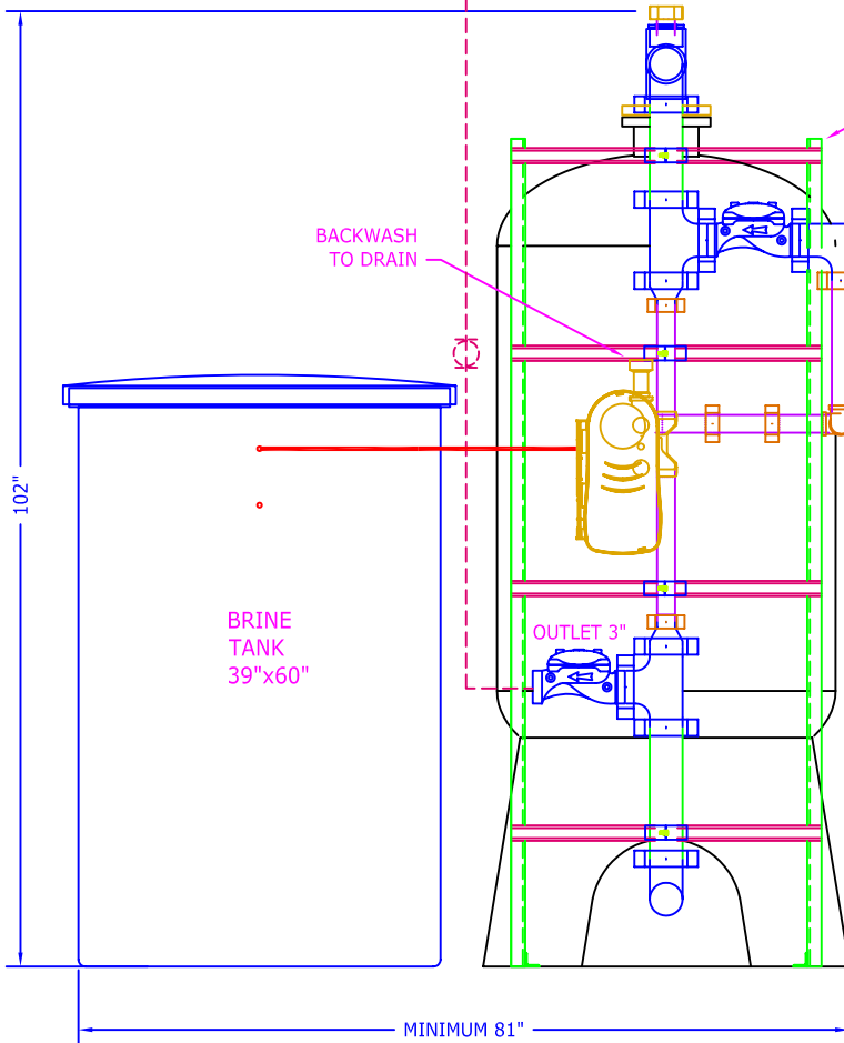
ELEVATION
