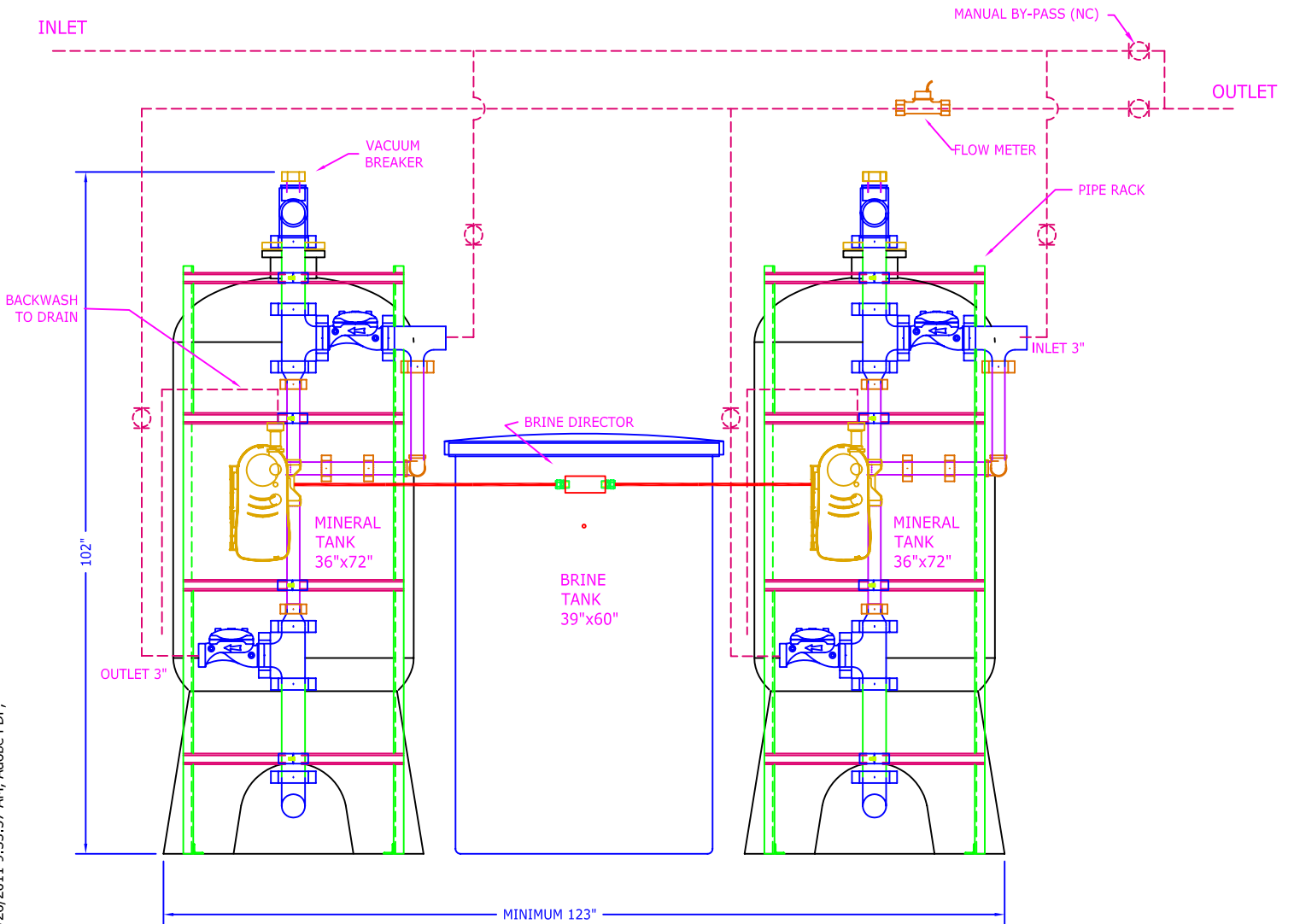
ELEVATION
