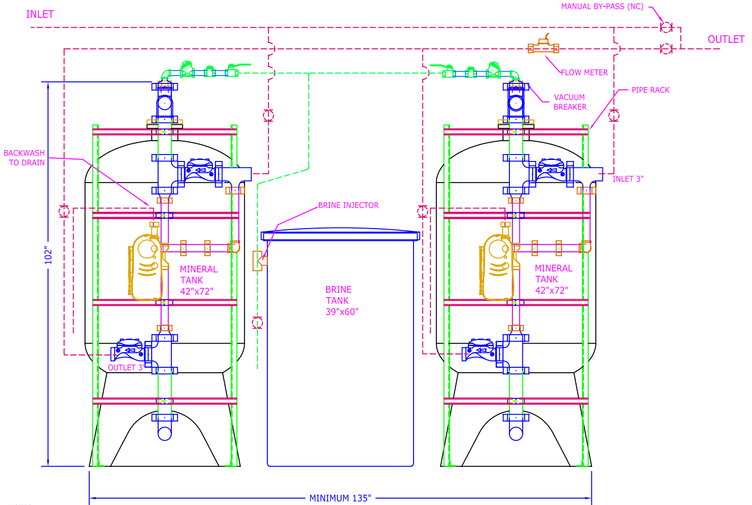
ELEVATION
