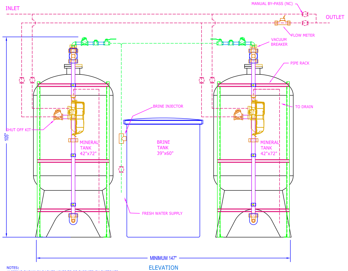
ELEVATION
