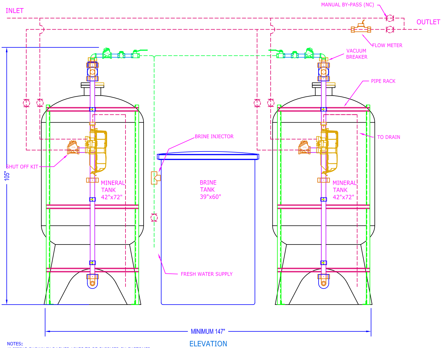
ELEVATION
