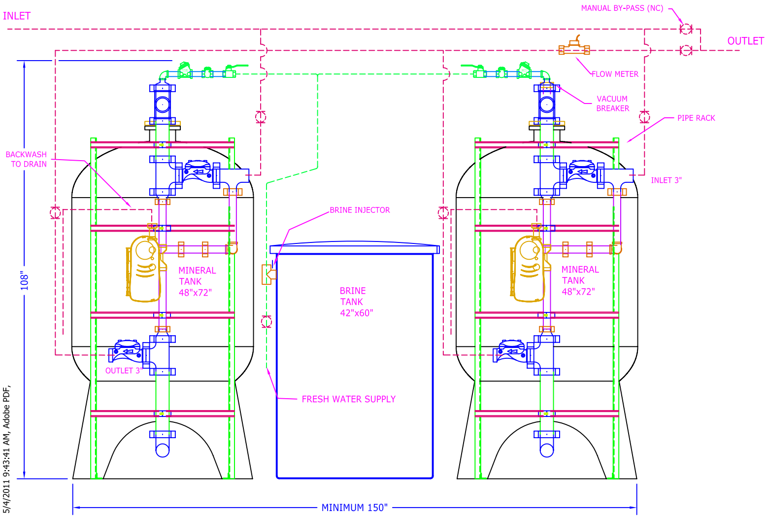
ELEVATION
