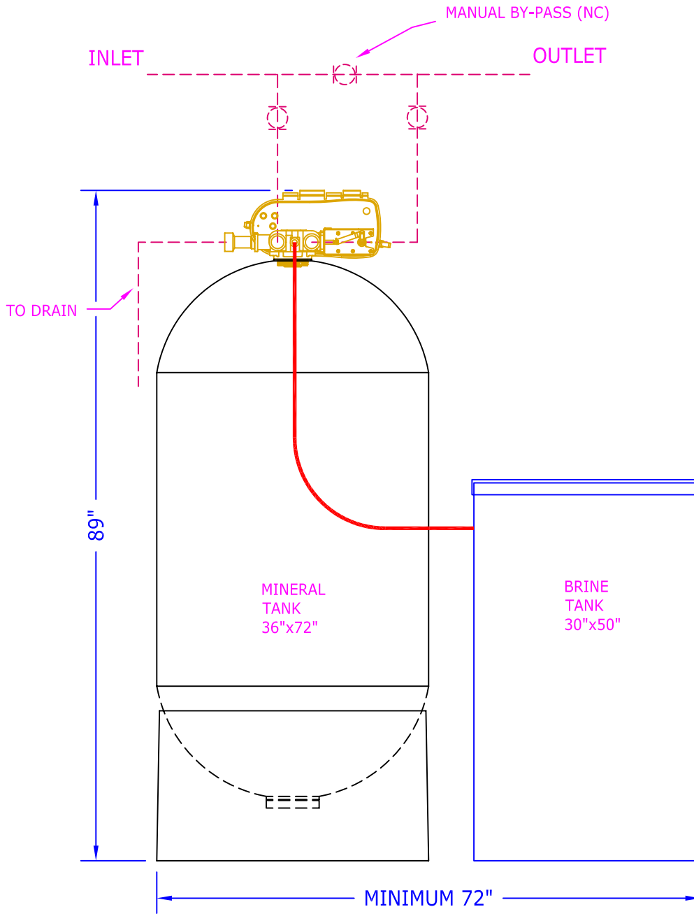
ELEVATION
