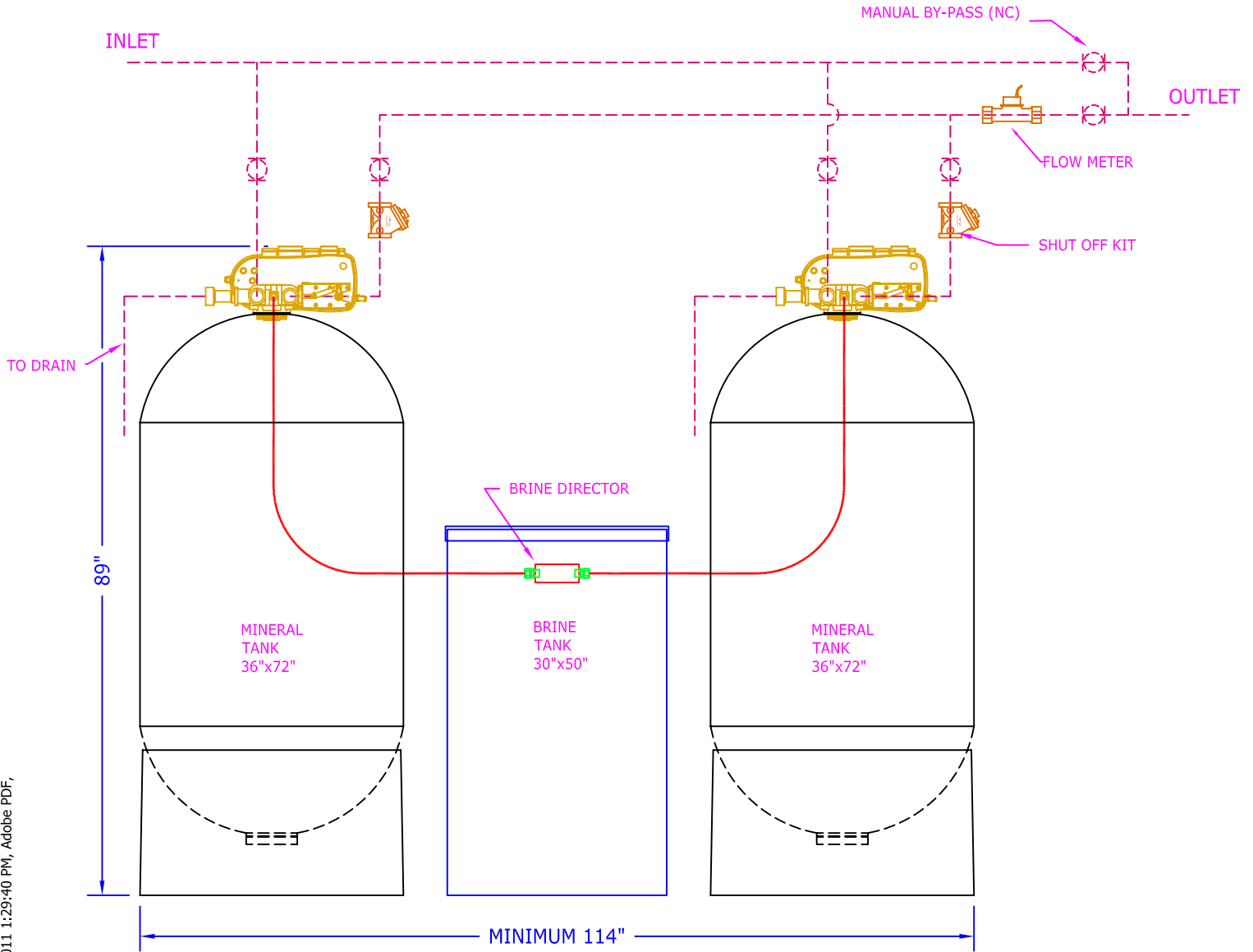
ELEVATION
