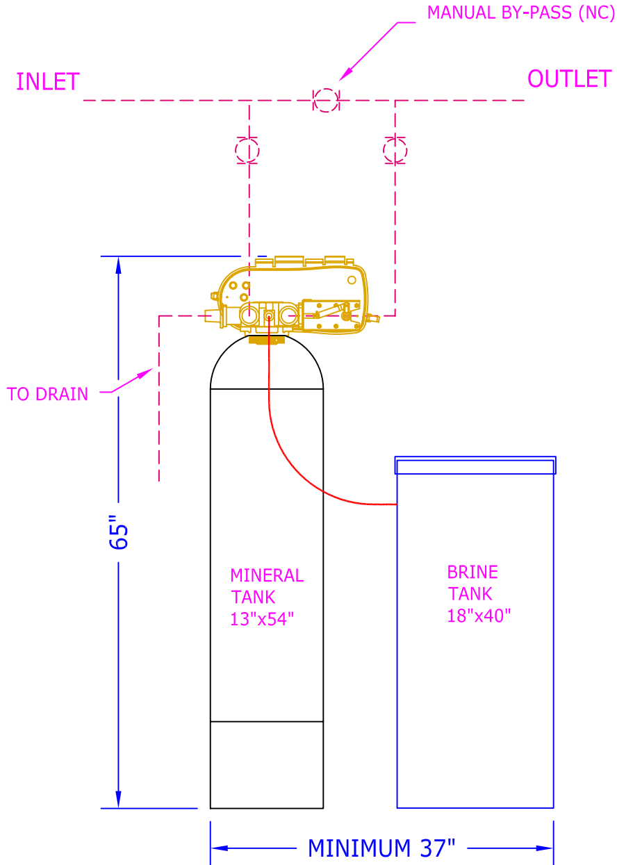
ELEVATION
