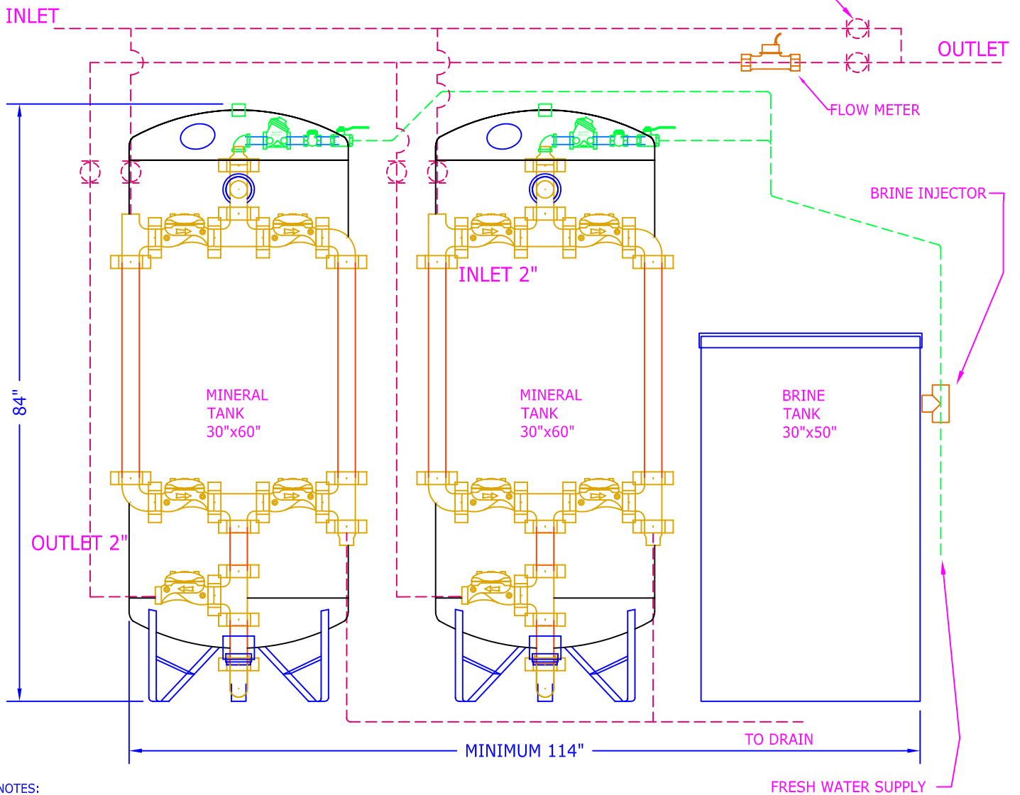
ELEVATION
