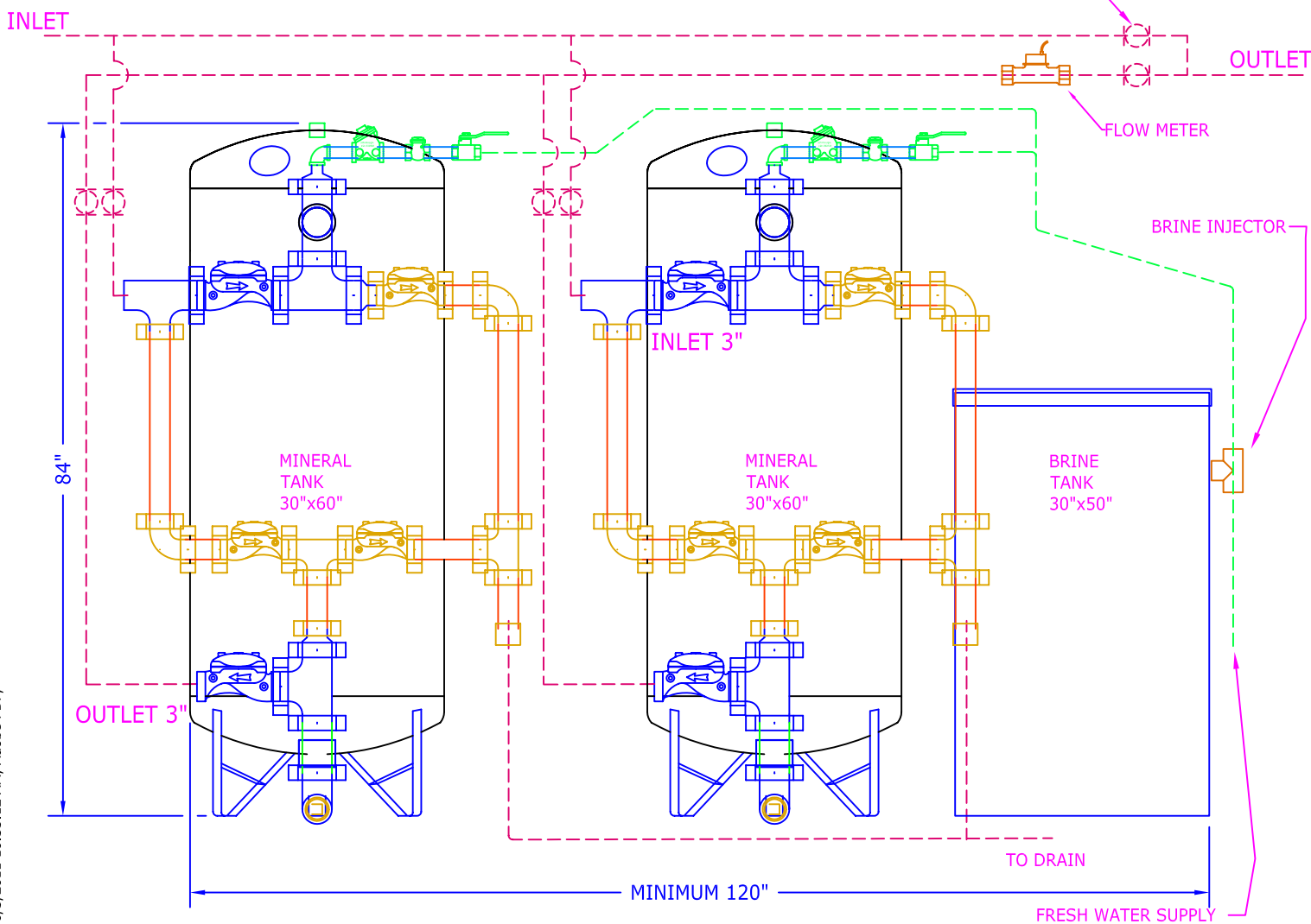
ELEVATION
