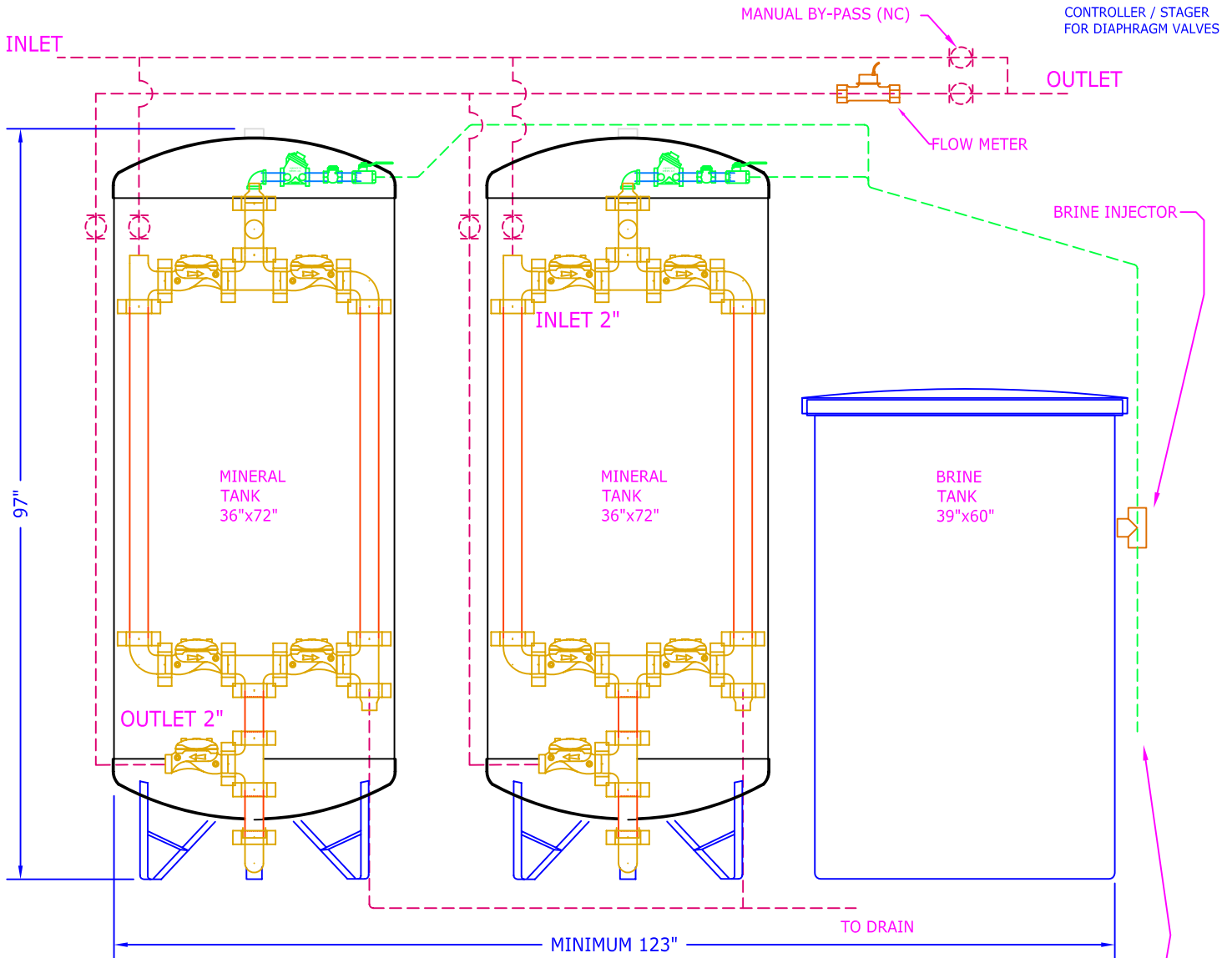
ELEVATION
